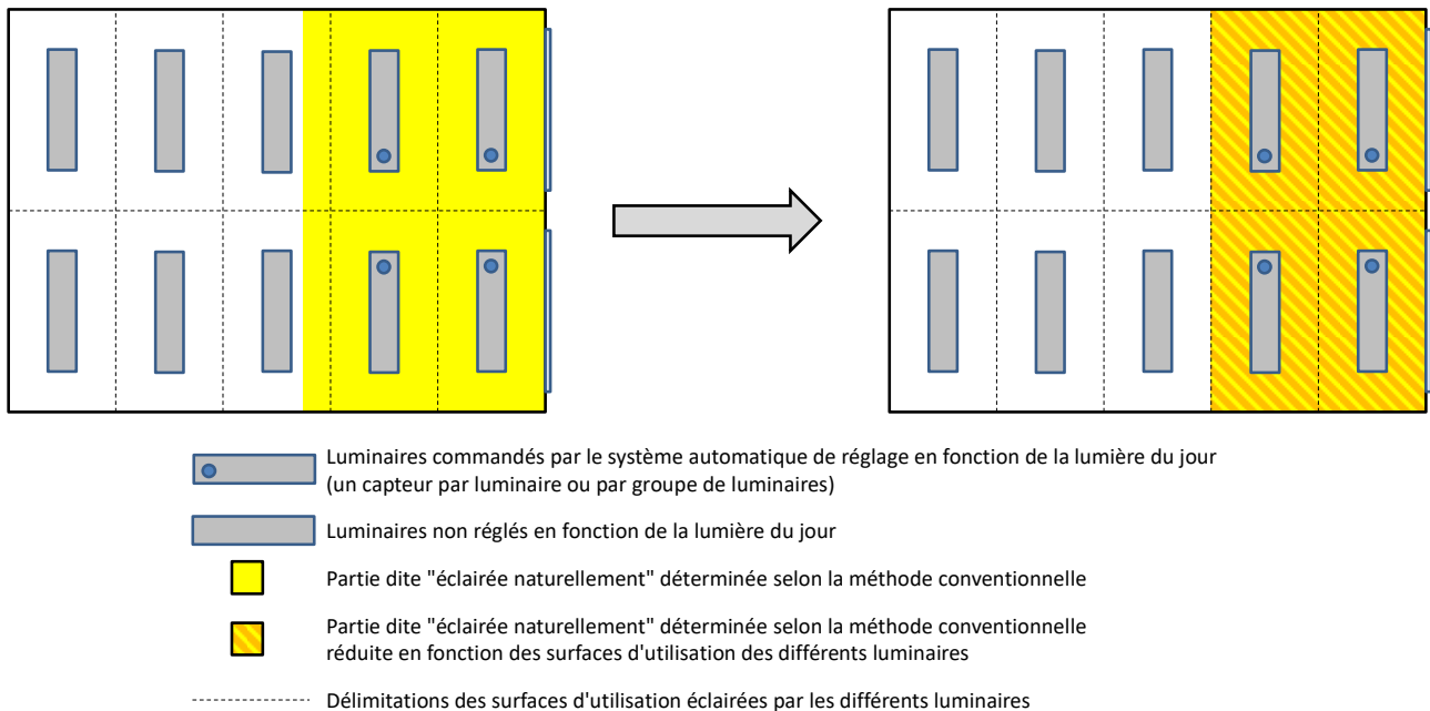
Abbildung [3]: Konfiguration, bei der die berücksichtigten Leuchten nicht von demselben System gesteuert werden - die sogenannte „tageslichtbeleuchtete“ Fläche befindet sich teilweise außerhalb der vom System gesteuerten Gesamtnutzfläche
