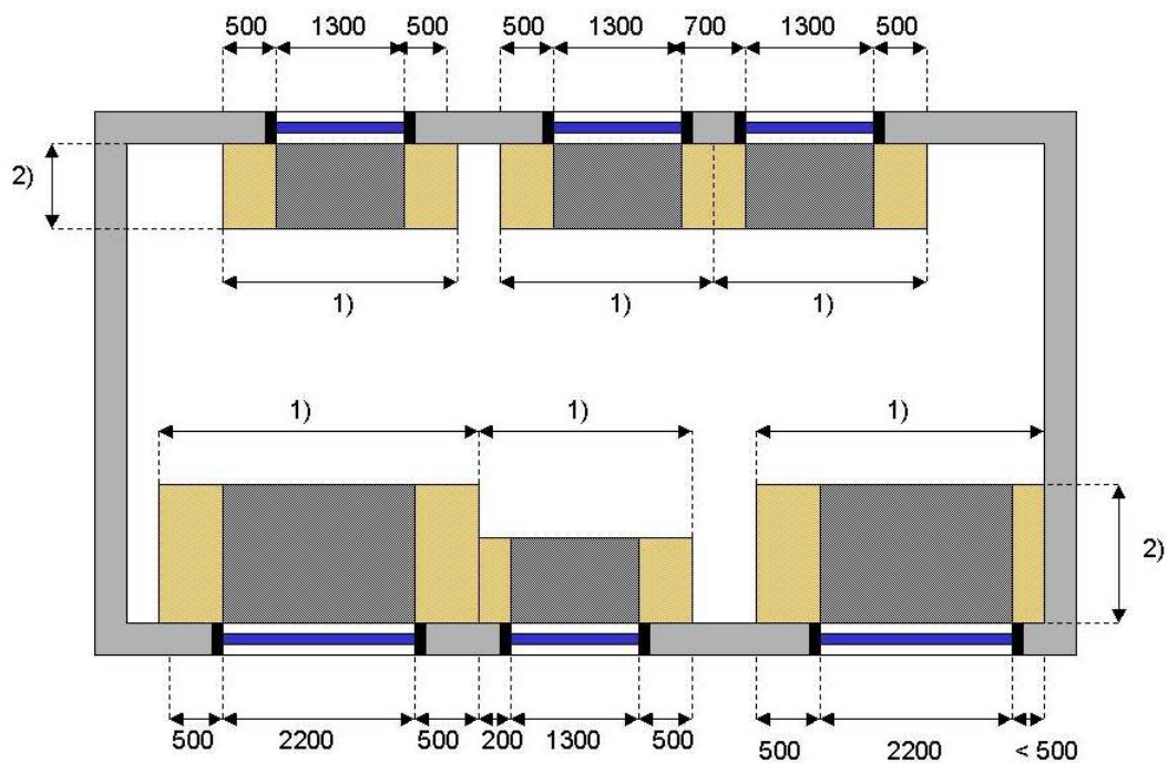
Abbildung [6]: Bereiche der Nutzfläche hinter lichtdurchlässigen und lichtundurchlässigen Elementen einer Fassade, die zum sogenannten „tageslichtbeleuchteten“ Bereich gehören
