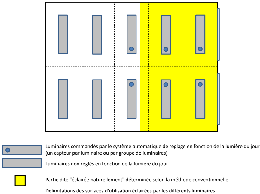
Abbildung [2]: Konfiguration, bei der die berücksichtigten Leuchten nicht von demselben System gesteuert werden - die sogenannte „tageslichtbeleuchtete“ Fläche befindet sich vollständig in der vom System gesteuerten Gesamtnutzfläche
